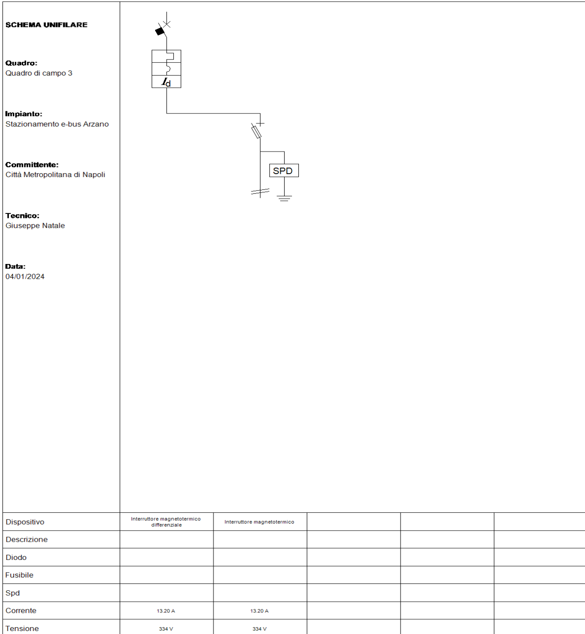
Fig. 8: Schema unifilare quadro "Quadro di campo 3"
