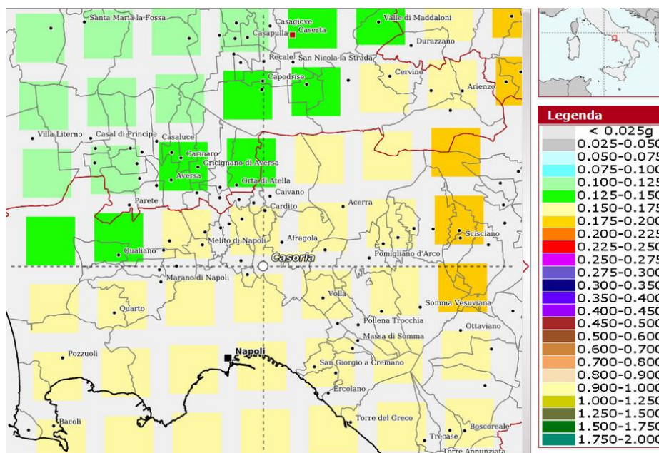
Mappa della pericolosità sismica del territorio comunale di Casoria (NA) dell'INGV con i range di valori delle ag nella legenda corrispondente
