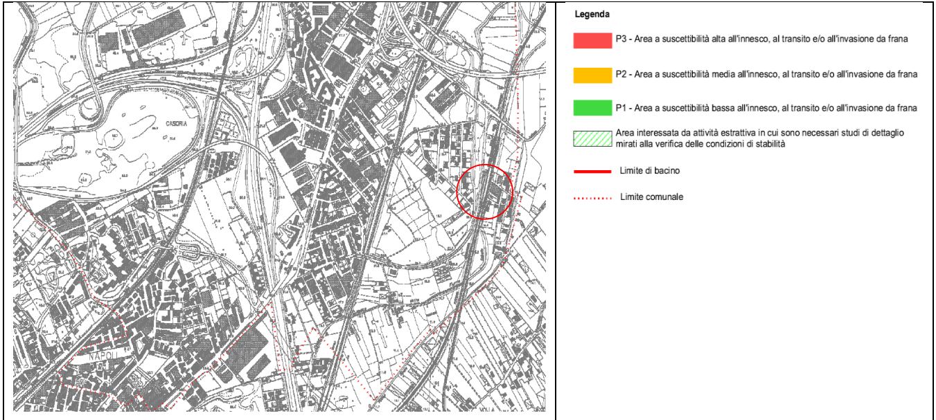
Stralcio della carta della pericolosità frane dell'Autorità di Bacino Nord Occidentale della Campania.
